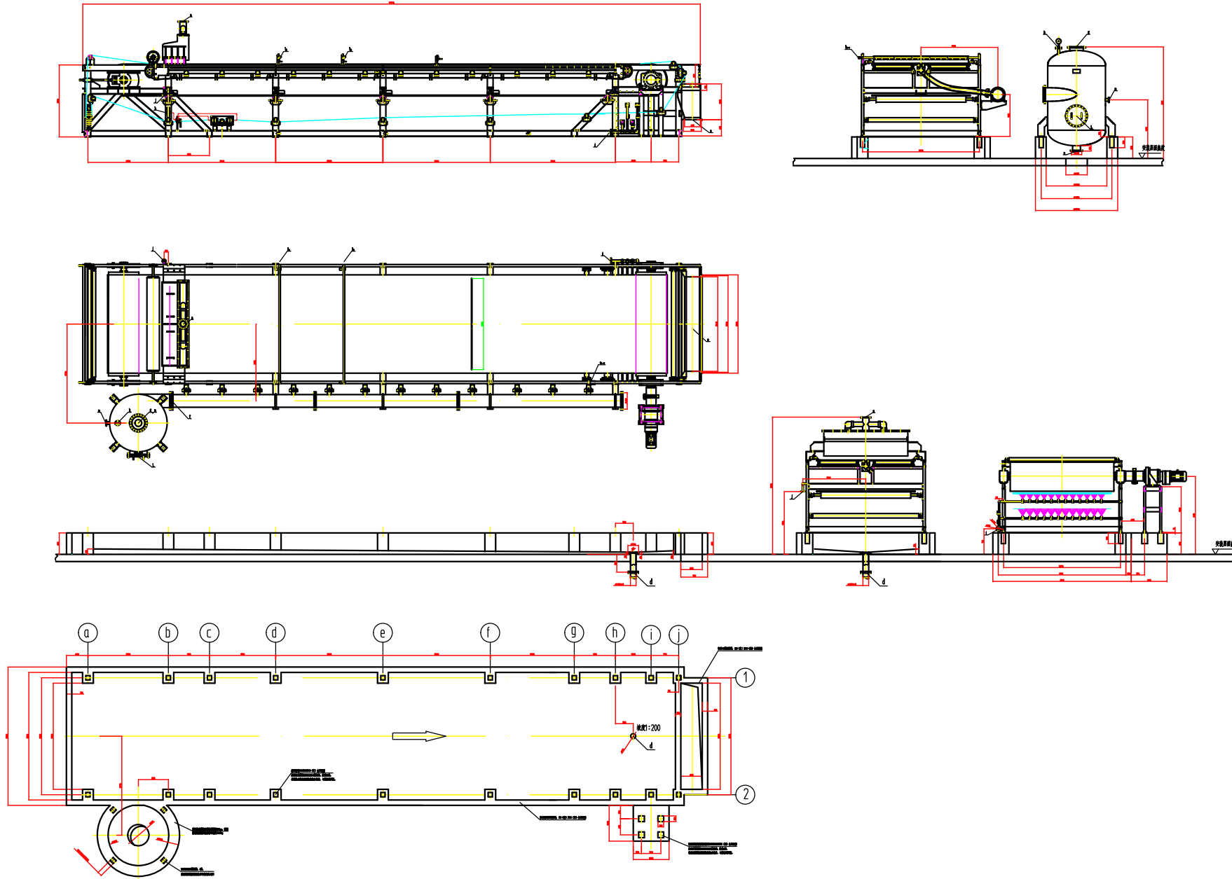
石膏脱水机及滤液收集罐基础尺寸图
